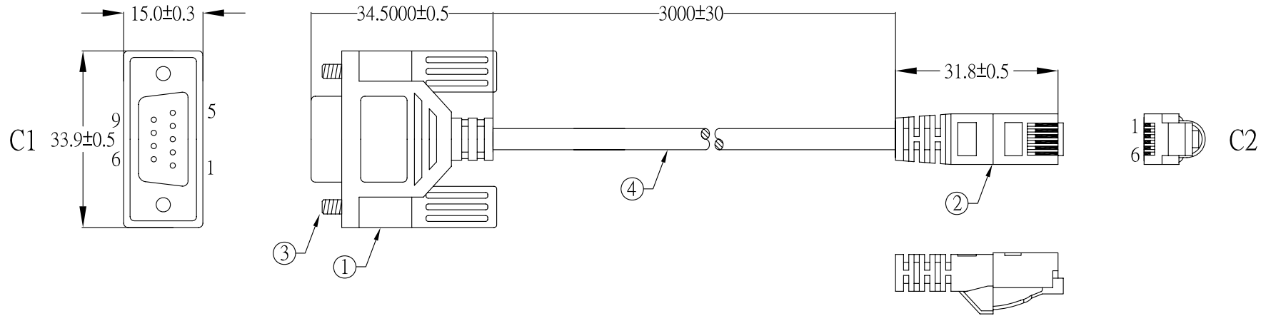
結線図
