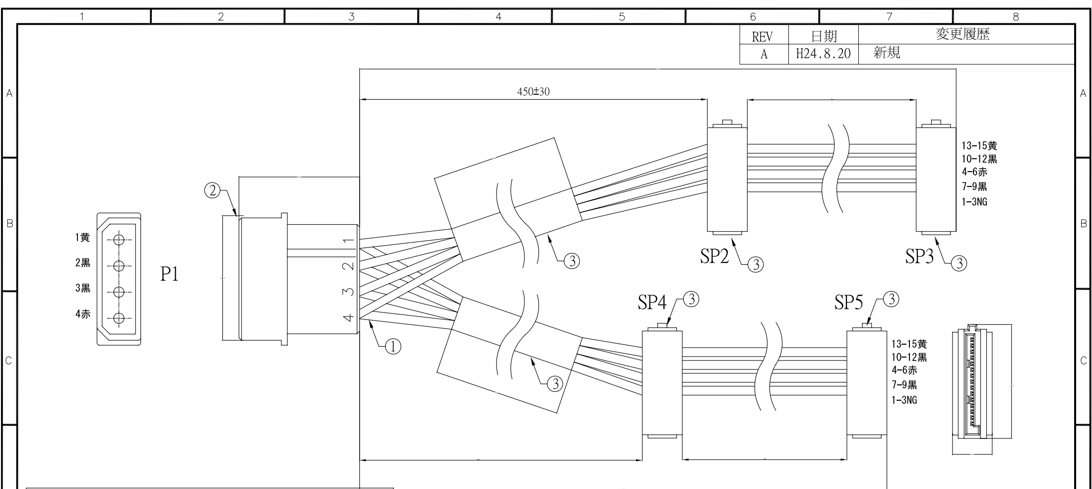
結線図
