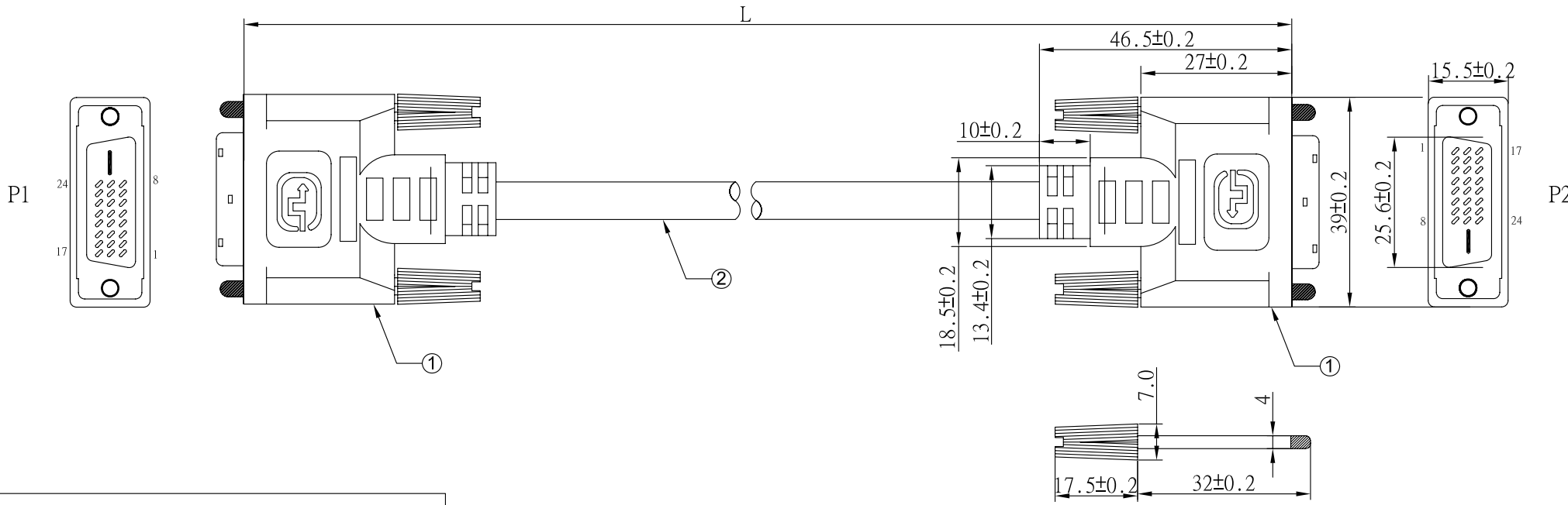
結線図
